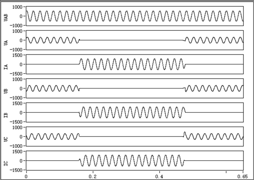
试 验 示 波 图
